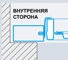
Ворота типа N80 Упор сзади проема
