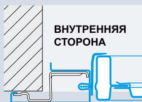
Ворота типа F80 Упор спереди проема
