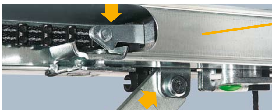
Устройство запирания ворот в приводной шине - патент Hörmann
