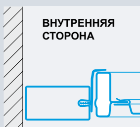
Ворота типа N80 Упор в проеме
